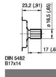
T1 Coppia Max Max Torque 130 Nm
