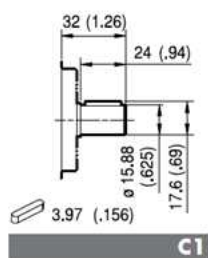
A Coppia Max Max Torque 105 Nm
