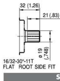
S2 Coppia Max Max Torque 230 Nm
