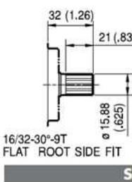
C1 Coppia Max Max Torque 110 Nm
