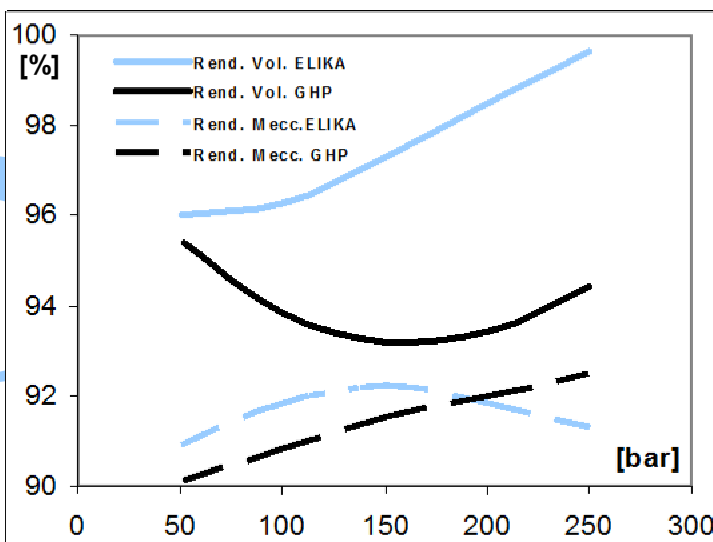
Confronto rendimenti [%] pompe Marzocchi GHP 2 – ELIKA ELI 2 di medesima cilindrata 17.8 cm 3 /giro., velocità 1500 giri/min.
