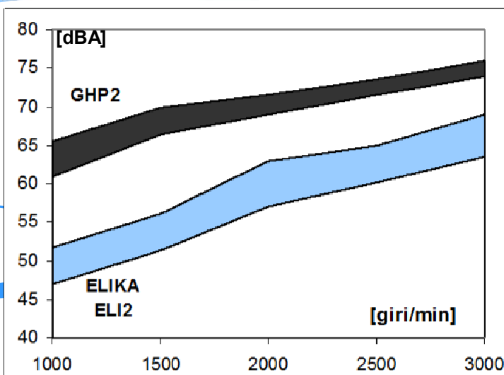
Confronto rumorosità [dBA] pompe Marzocchi GHP 2 – ELIKA ELI 2 di medesima cilindrata 17.8 cm 3 /giro, pressioni da 10 a 250 bar.
