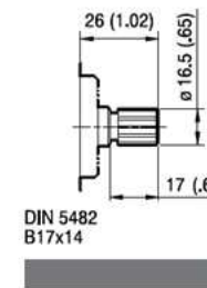
T2 Coppia Max Max Torque 130 Nm
